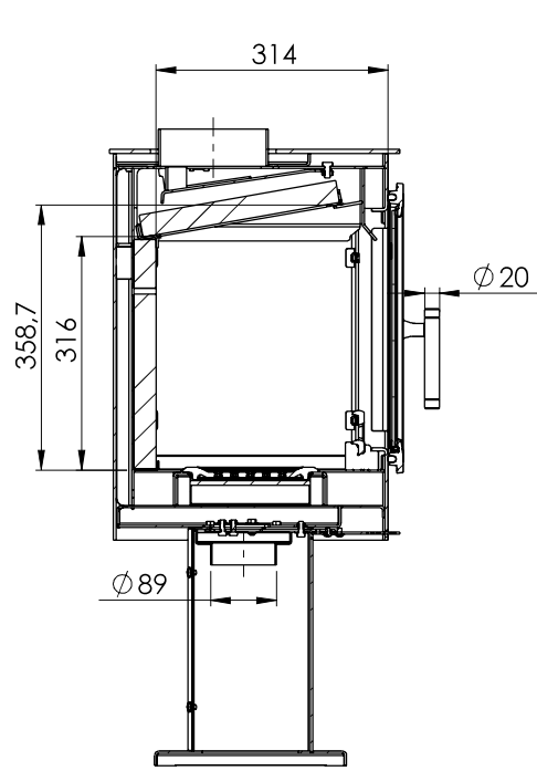
PRZEKRÓJ A-A SKALA 1 : 8
