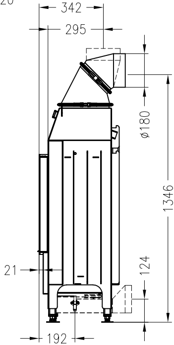
Seitenansicht
