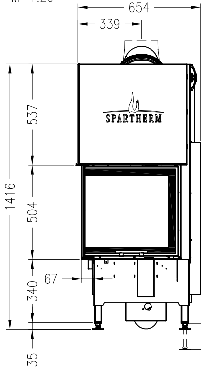
Vorderansicht M~1:20
