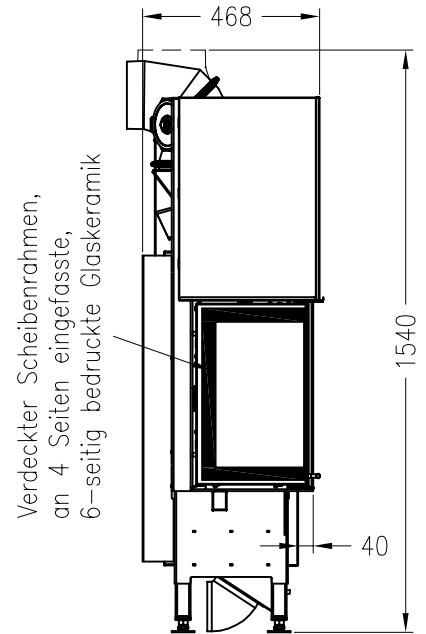
Seitenansicht M~1:20
